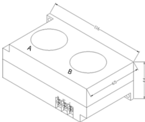
Рисунок 4.1.1. Габаритные размеры СТ1 СТ1
